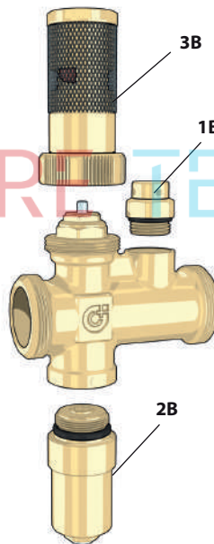
Nezámrzný ventil se senzorem vzduchu
