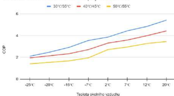
MONOBLOCK 12kW 3Ph - Topný faktor COP
