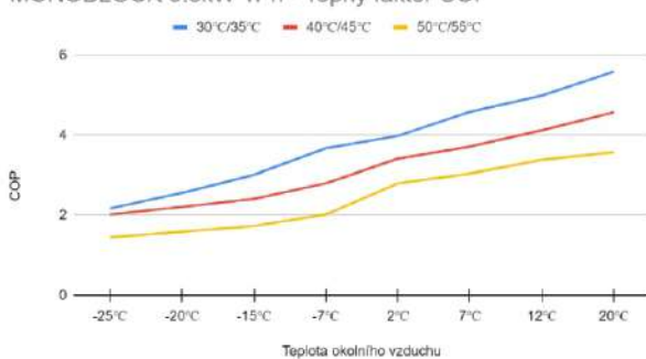
MONOBLOCK 9.5kW 1Ph - Topný faktor COP
