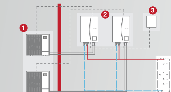
1 Vonkajšie jednotky 2 Hydromodul 3 PAC-IF071
